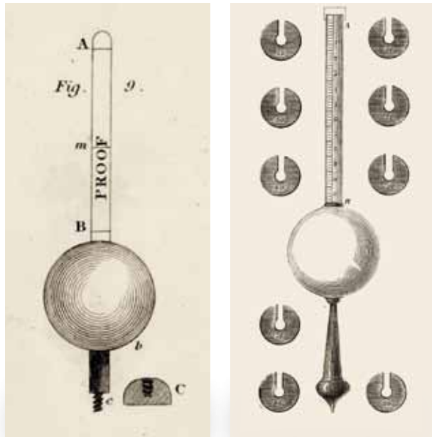
De hydrometer van Clarke.
